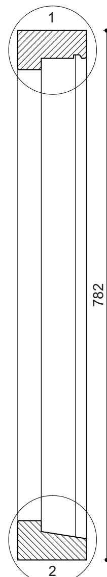
Doorsnede B-B
